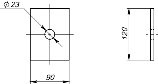
Поз.2 (Планка)
